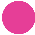
RHODAMINE
